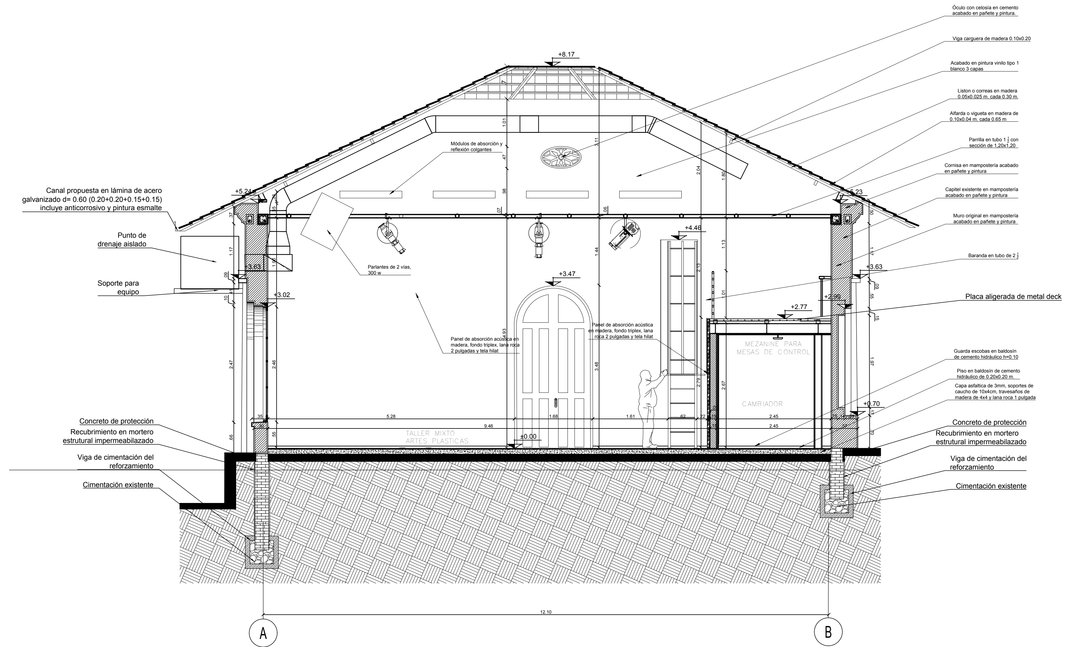
C2 CORTE B-B - PROPUESTA ESCALA 1:25
