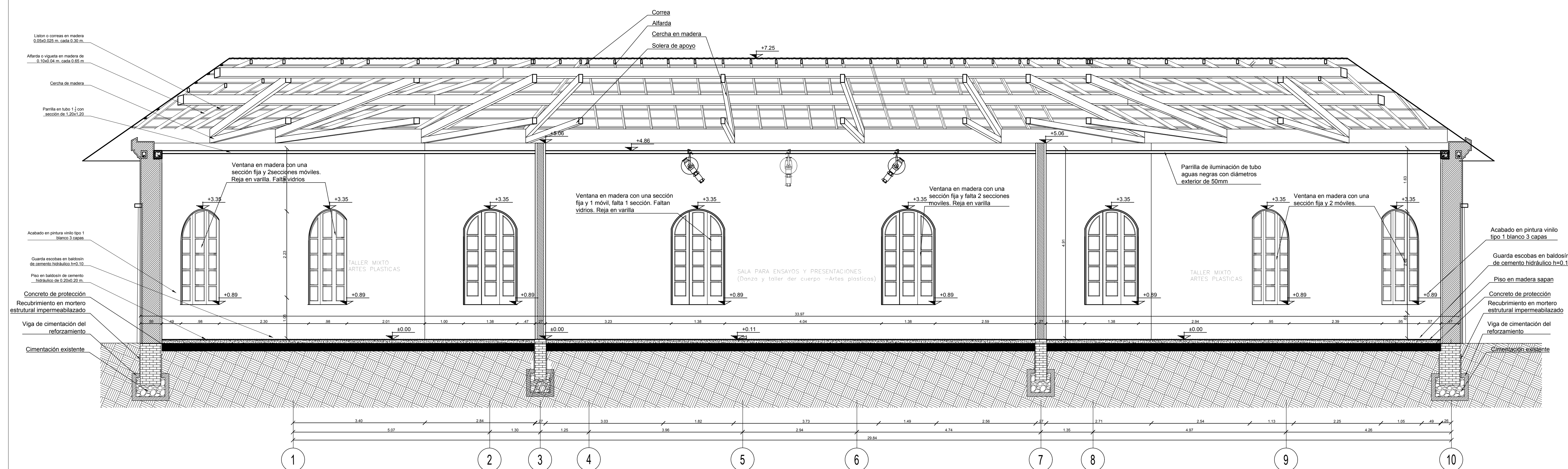
C5 CORTE D-D - PROPUESTA ESCALA 1:25
