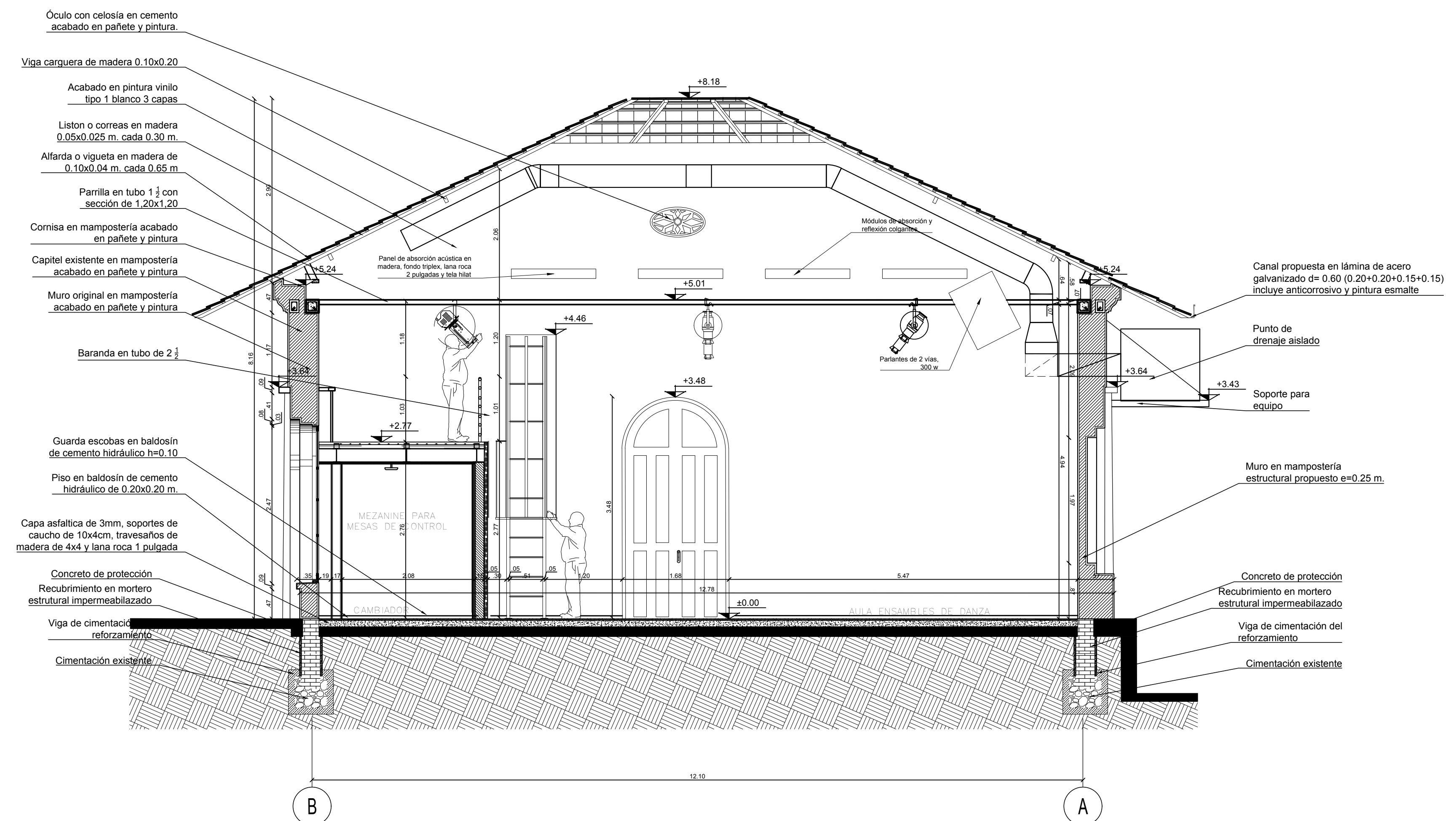
C3 CORTE C-C - PROPUESTA ESCALA 1:25
