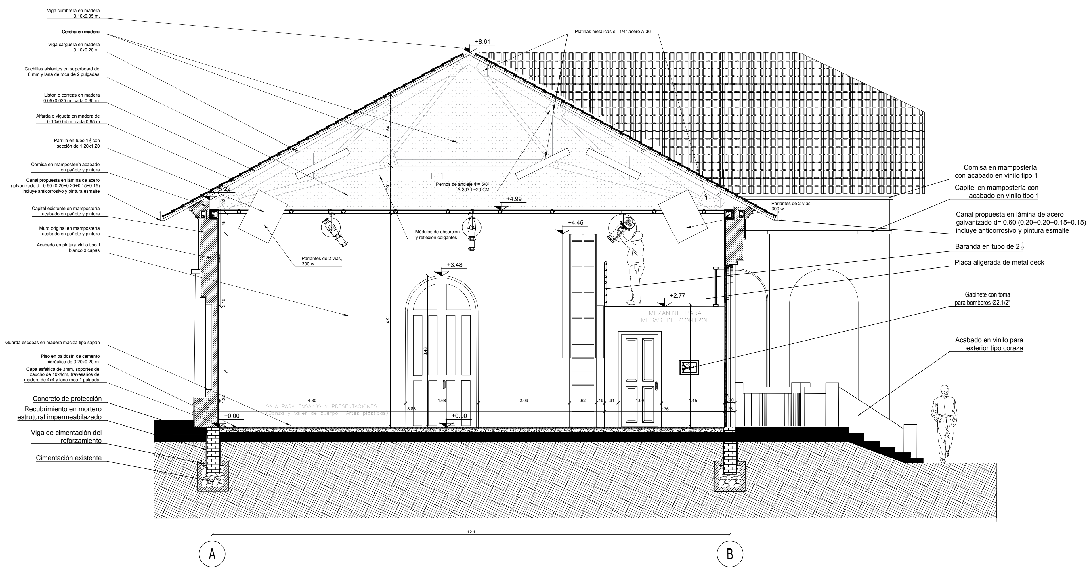
C1 CORTE A-A - PROPUESTA ESCALA 1:25
