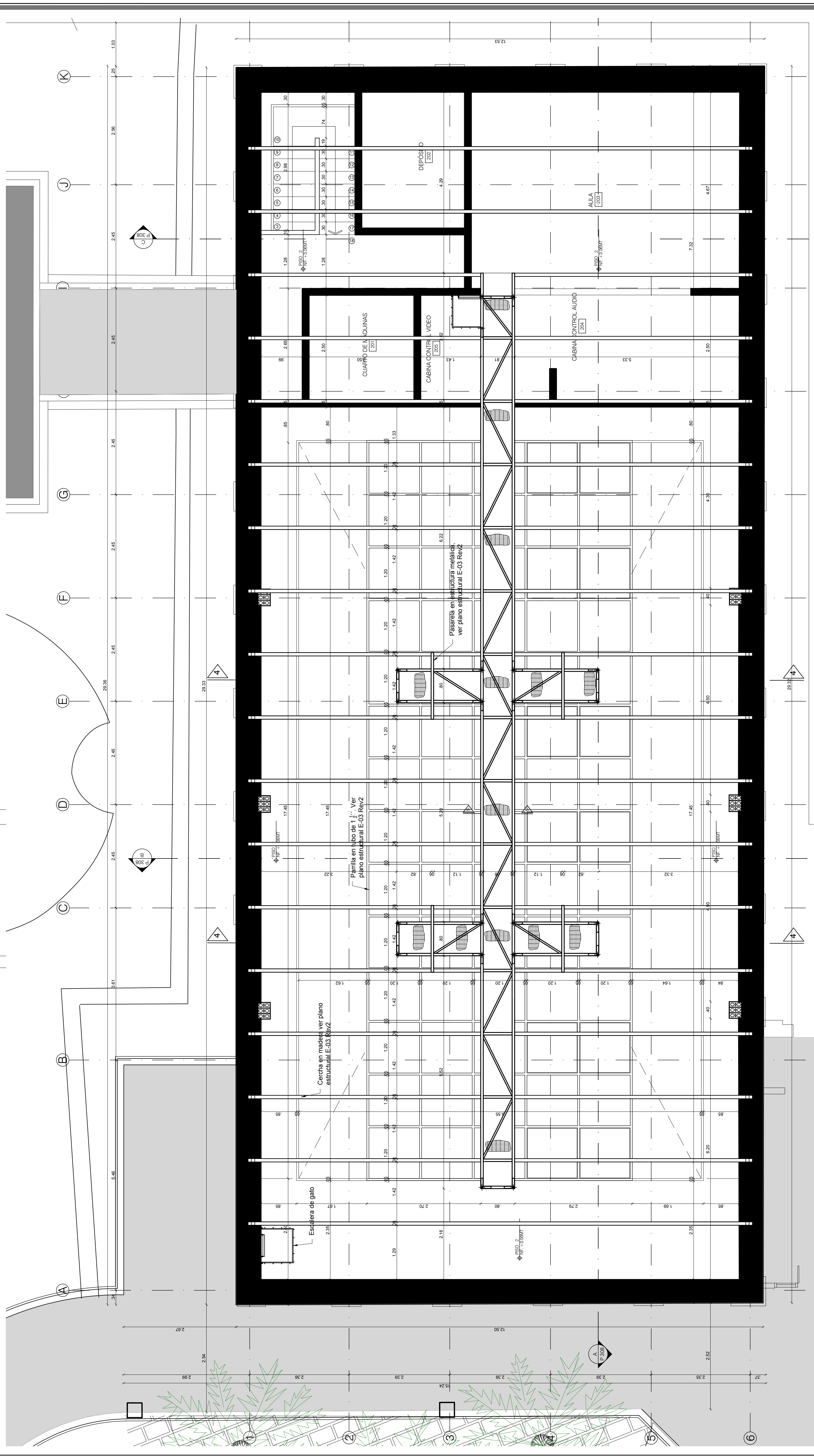
P2 PLANTA NIVEL PASARELA - PROPUESTA
