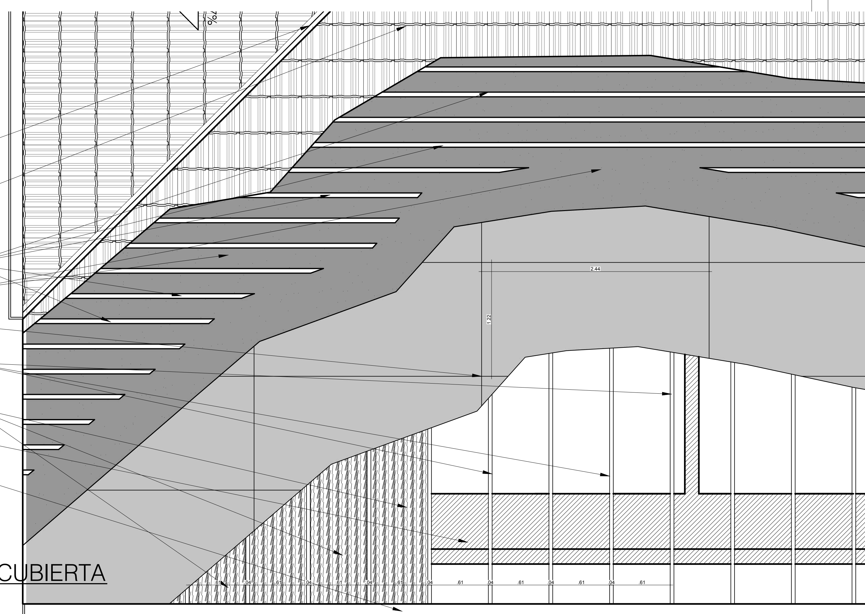
305 CORTE DETALLE CUBIERTA ESCALA 1:5
