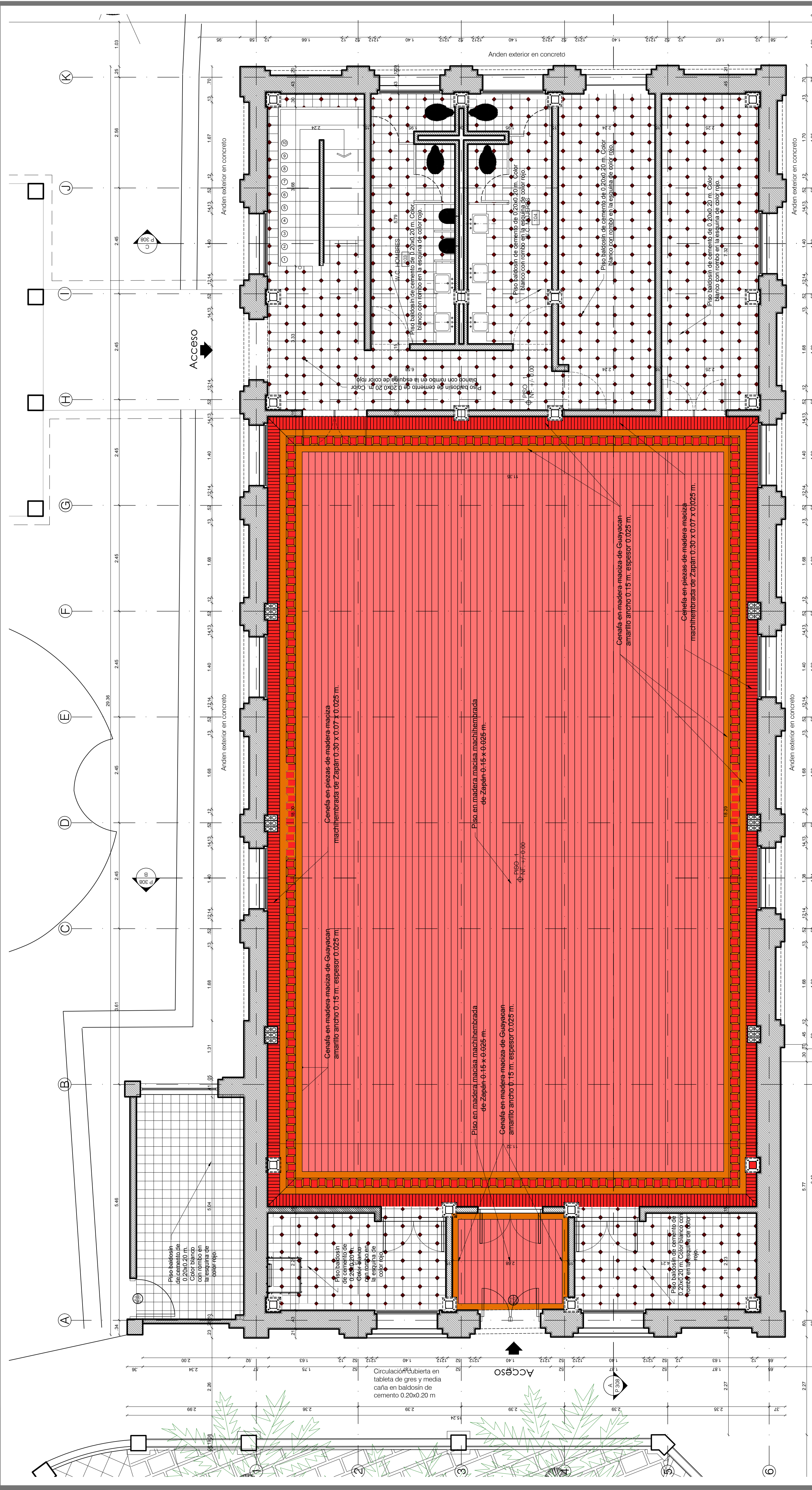
P1 PISOS PRIMER PISO - PROPUESTA ESCALA 1:50
