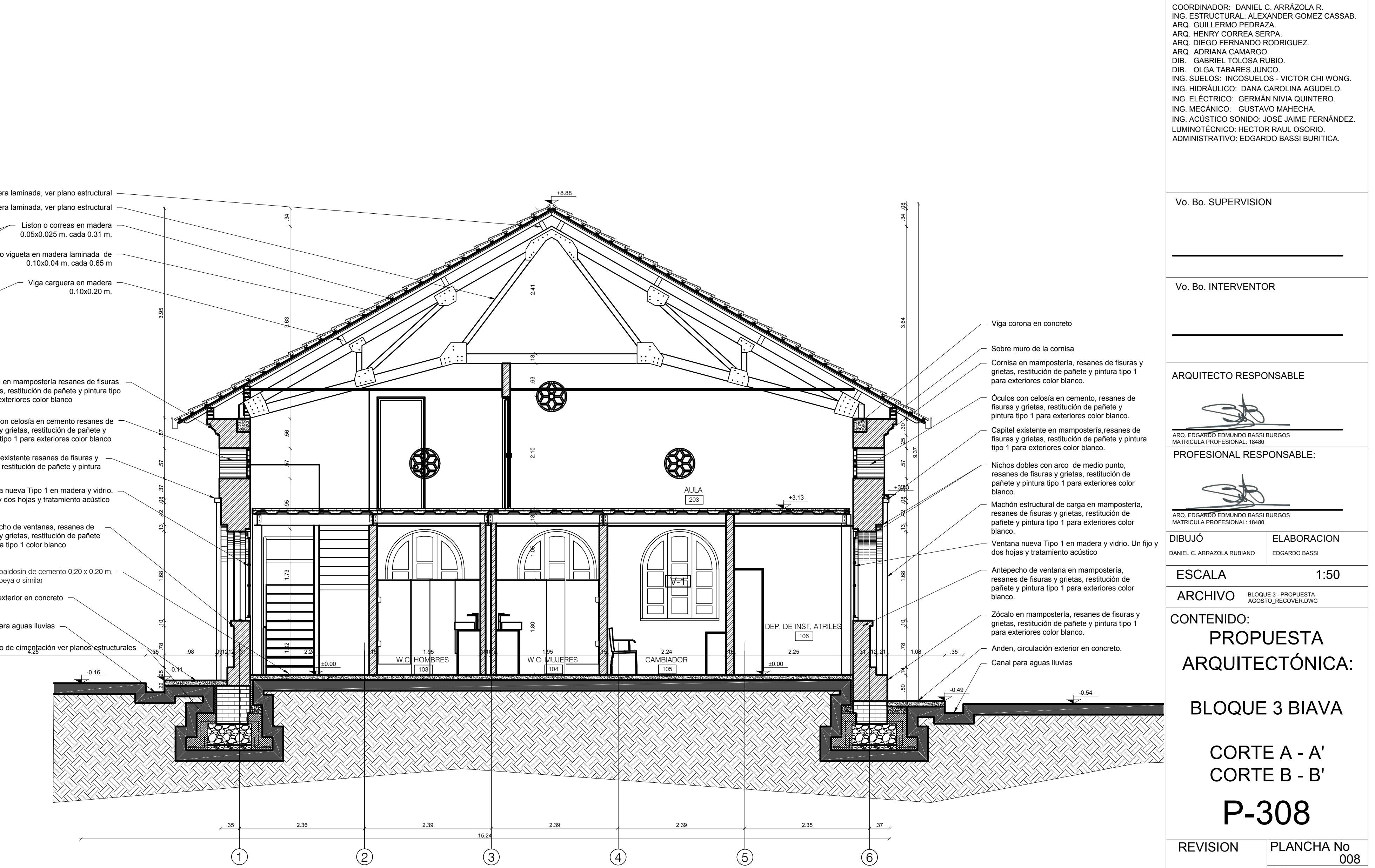
C1 CORTE A-A' - PROPUESTA ESCALA 1:50
