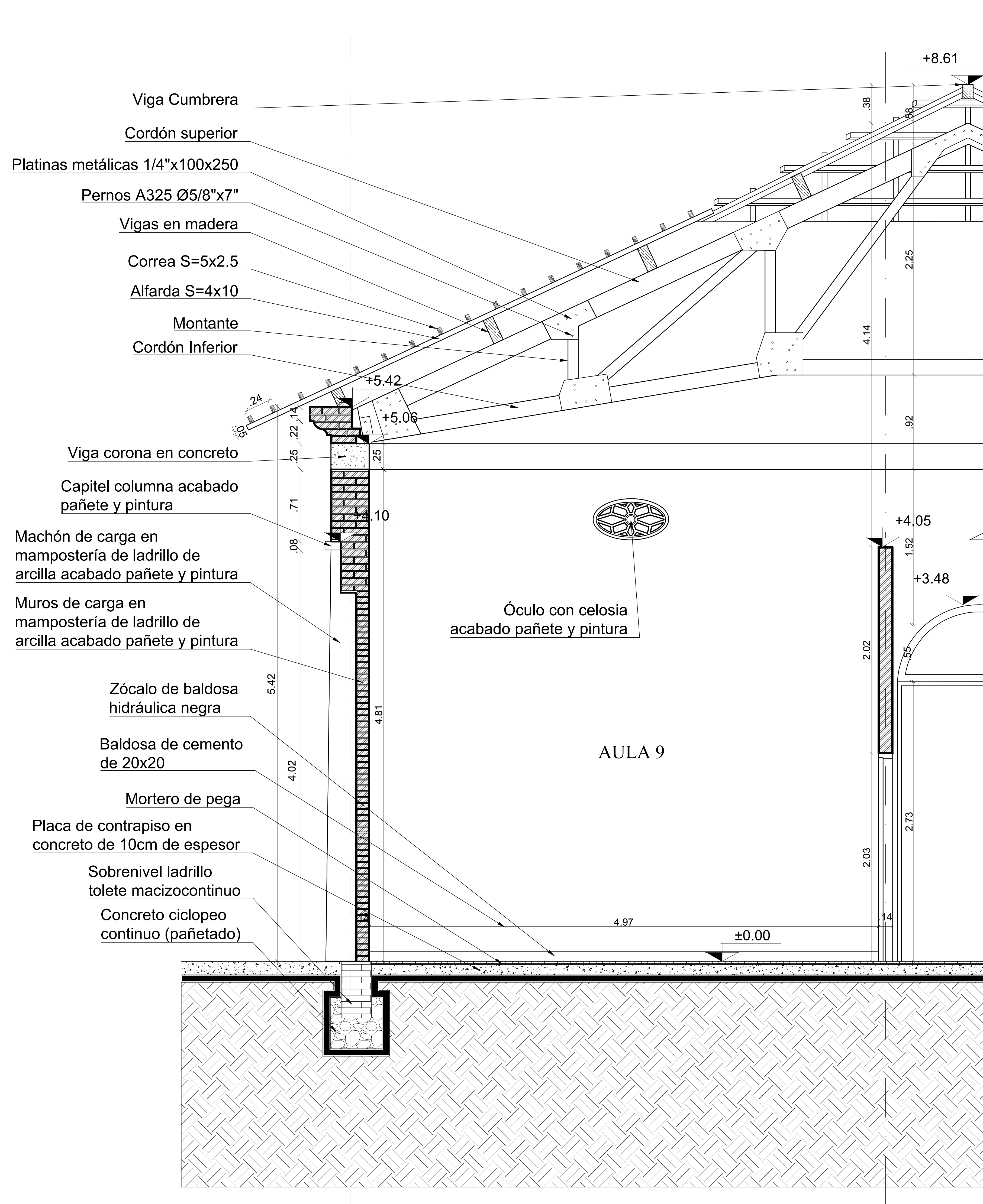
C2 CORTE FACHADA - LEVANTAMIENTO ESCALA 1:50
