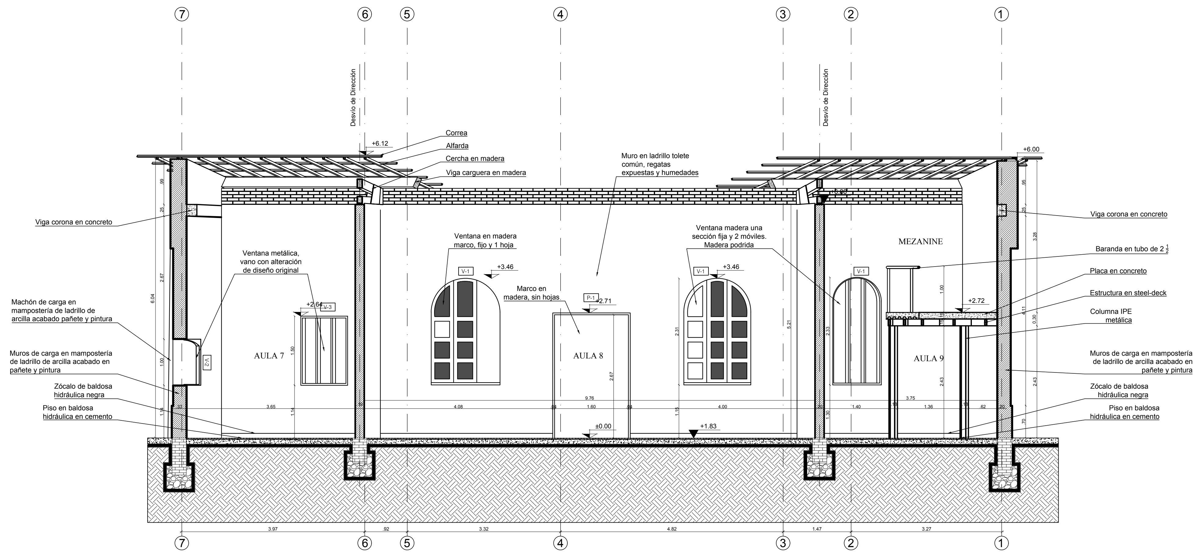
C3 CORTE C - C' - LEVANTAMIENTO ESCALA 1:50
