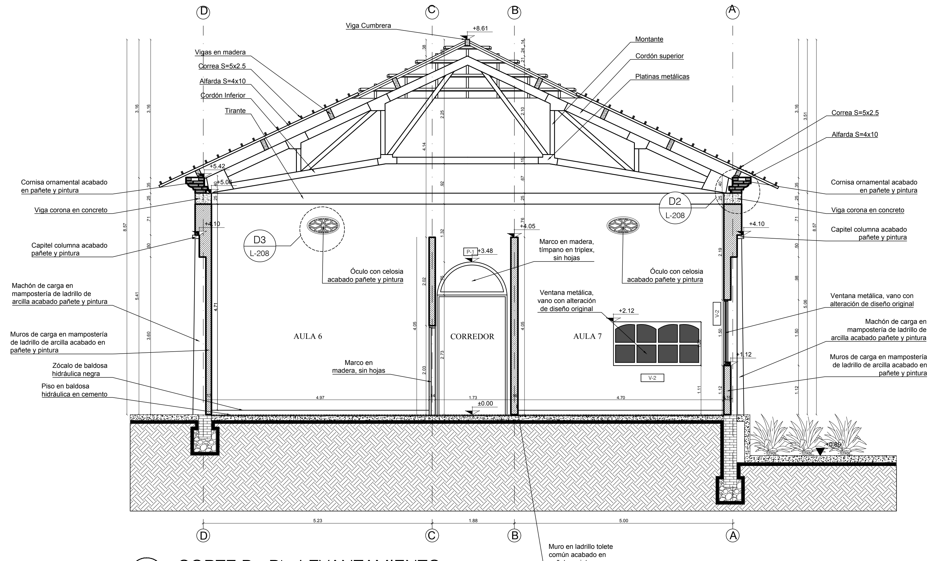
C2 CORTE B - B' - LEVANTAMIENTO ESCALA 1:50
