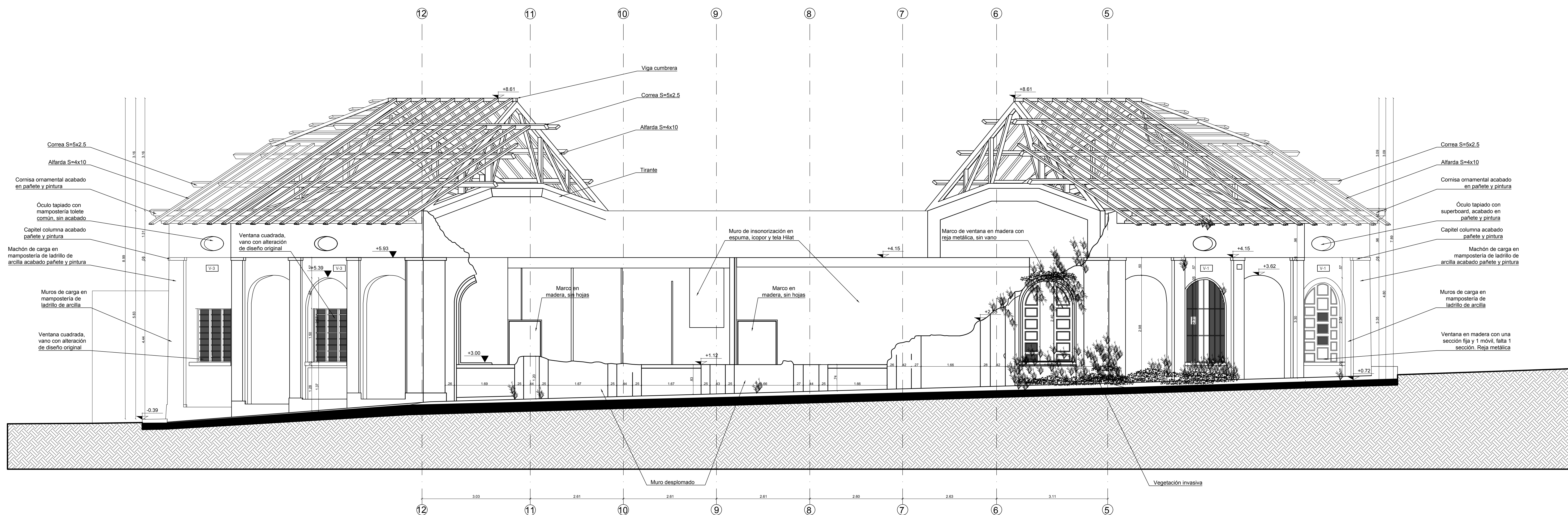
F3 FACHADA NORTE - LEVANTAMIENTO ESCALA 1:50
