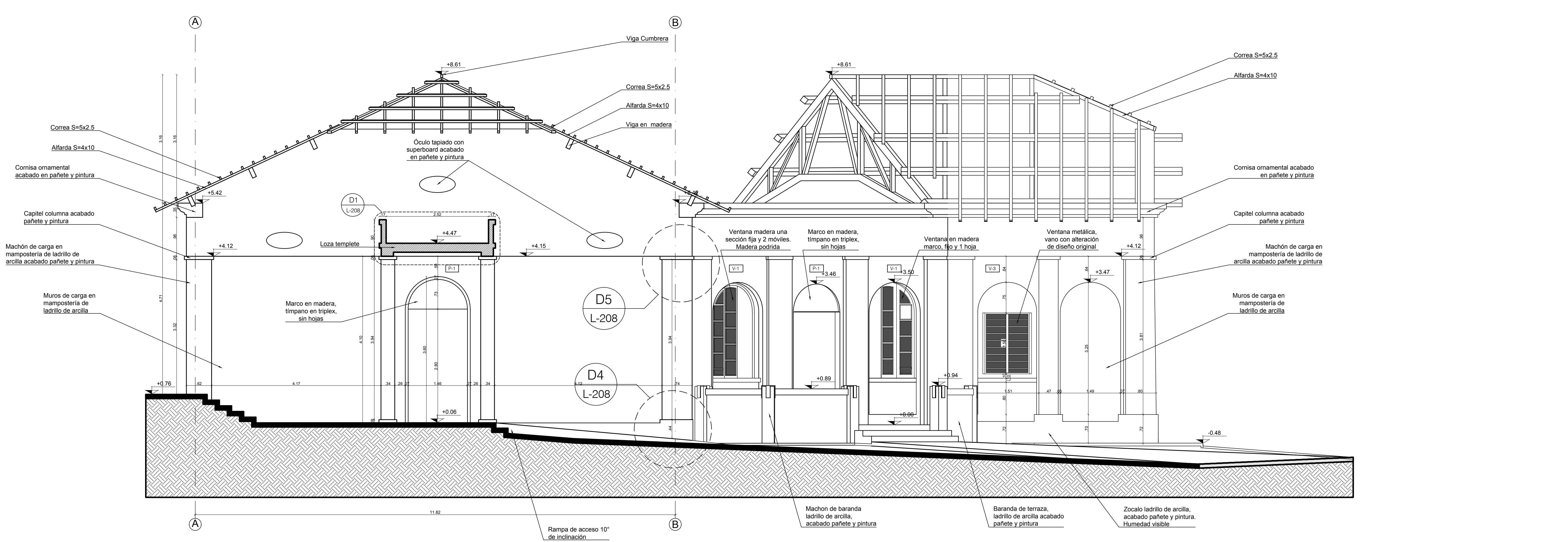
F2 FACHADA OESTE-LEVANTAMIENTO ESCALA 1:50
