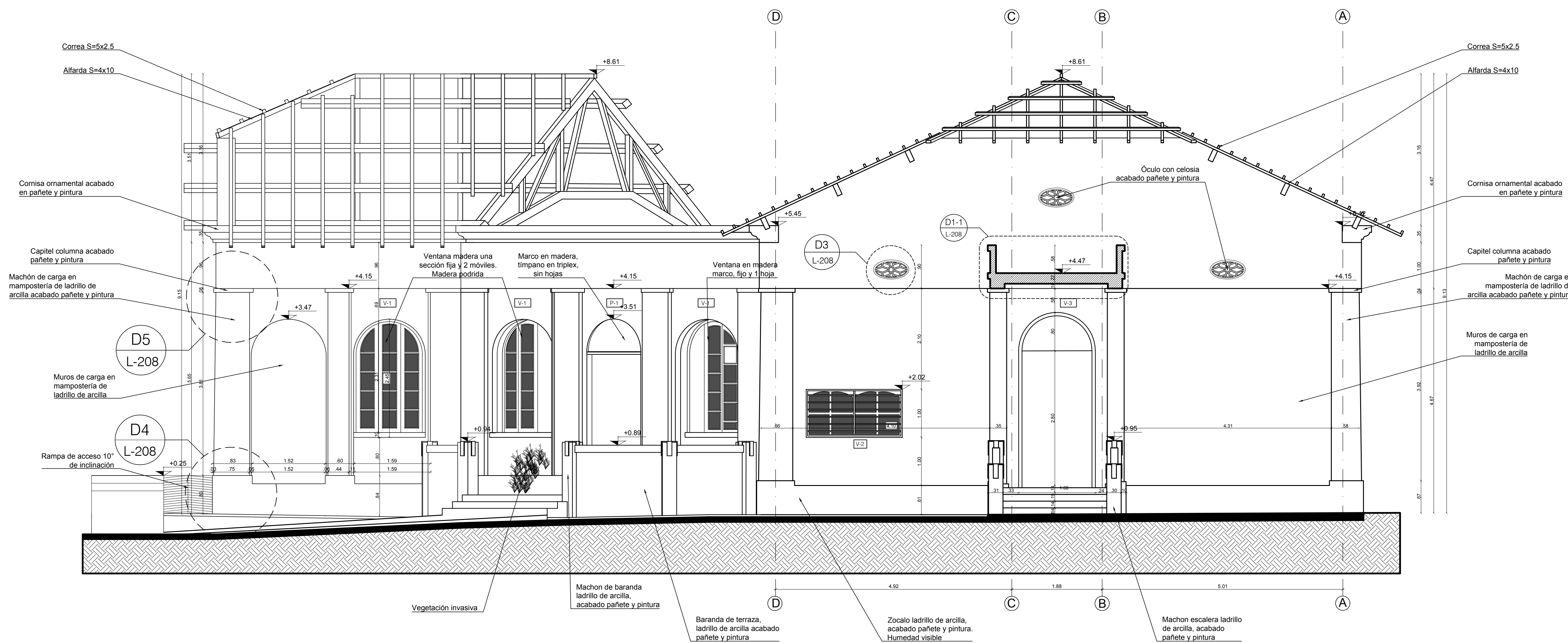
F4 FACHADA ESTE - LEVANTAMIENTO ESCALA 1:25
