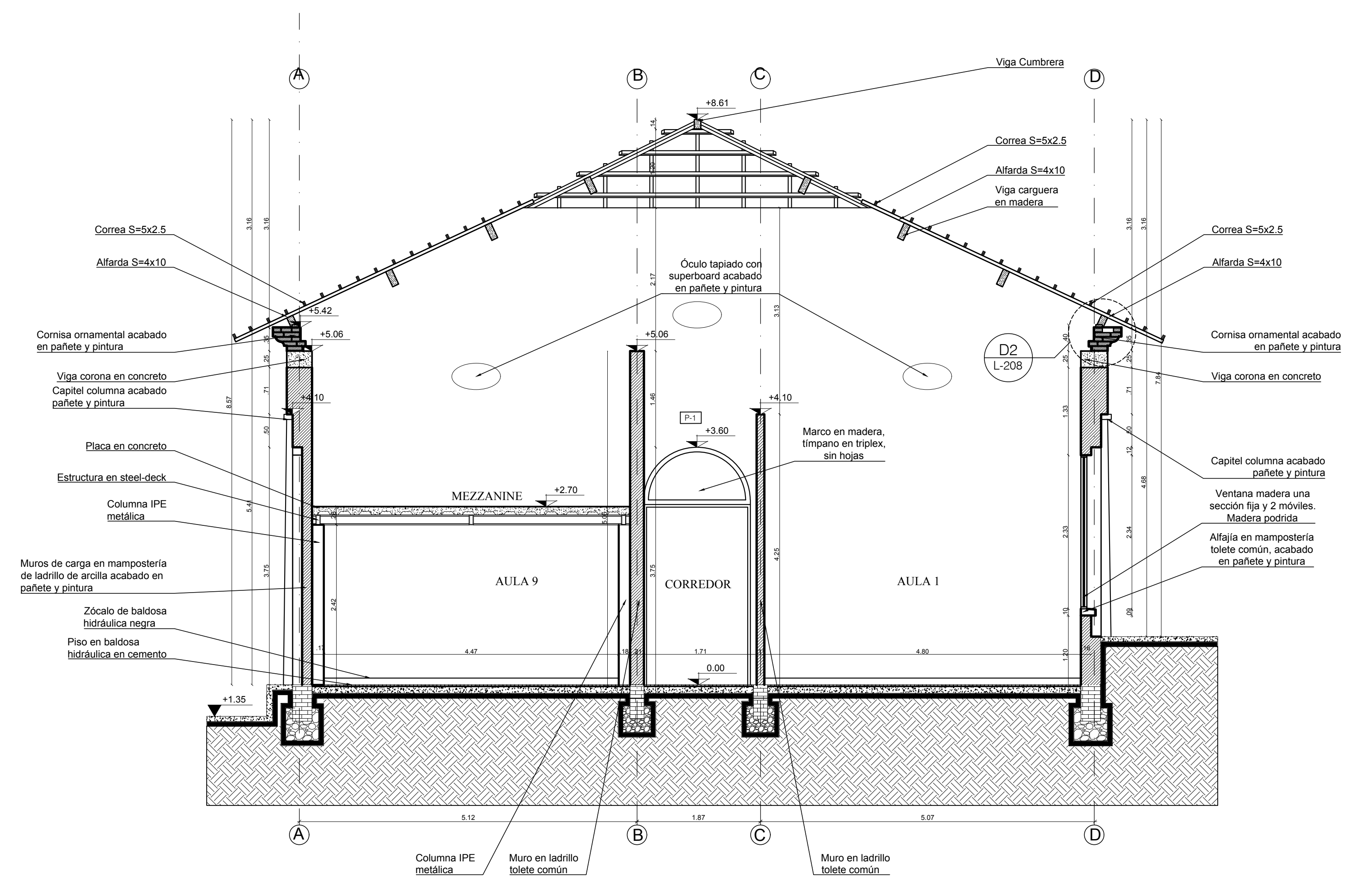
C1 CORTE A - A' - LEVANTAMIENTO ESCALA 1:50
